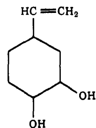
4 -Vinylcyclohexene-1,2-glycol
