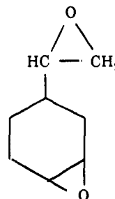
4 -Vinylcyclohexene diepoxide (4 -Epoxyethyl-1,2-epoxycyclohexane)
