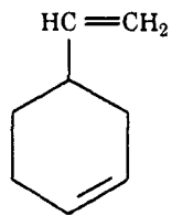
4 -Vinylcyclohexene
