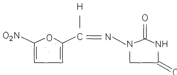
Nitrofurantoin
