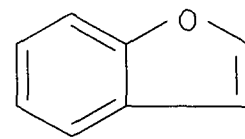
Benzofuran
